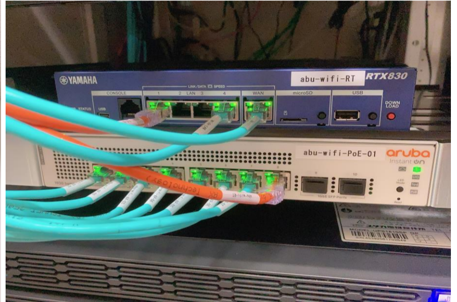
WiFiルーターLANケーブル配線(役場本庁電算室)
