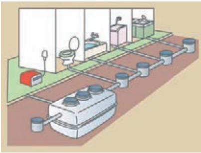
合併処理浄化槽 (環境省Webサイト)
